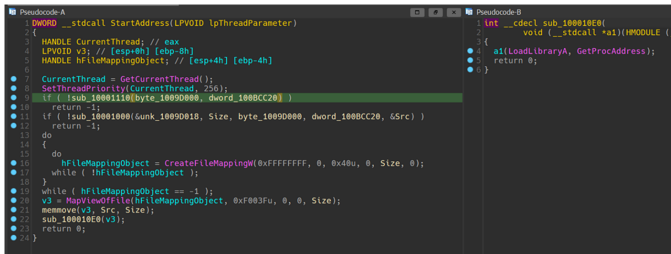
圖四、mpsvc.dll 使用 CreateFileMappingW 和 VirtualAllocEx 函式載入惡意程式核心
